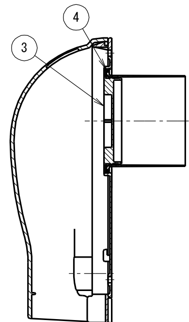
A-A断面
